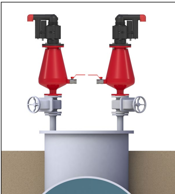
Dos ventosas sobre una trampa de aire con llaves de cierre separadas. Las salidas de las ventosas se dirigen hacia fuera y las llaves de cierre a 45° de las salidas de las ventosas
